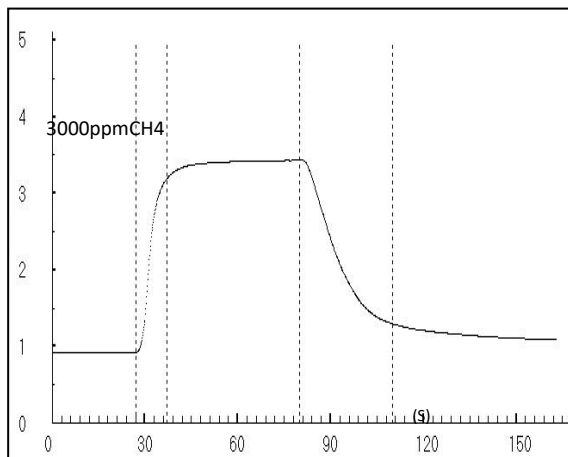
图 5: 响应恢复曲线图
