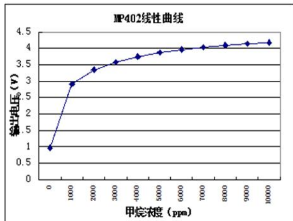
6: 传感器线性曲线
