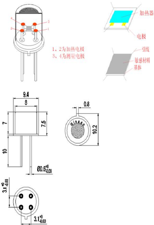
1: 传感器结构图
