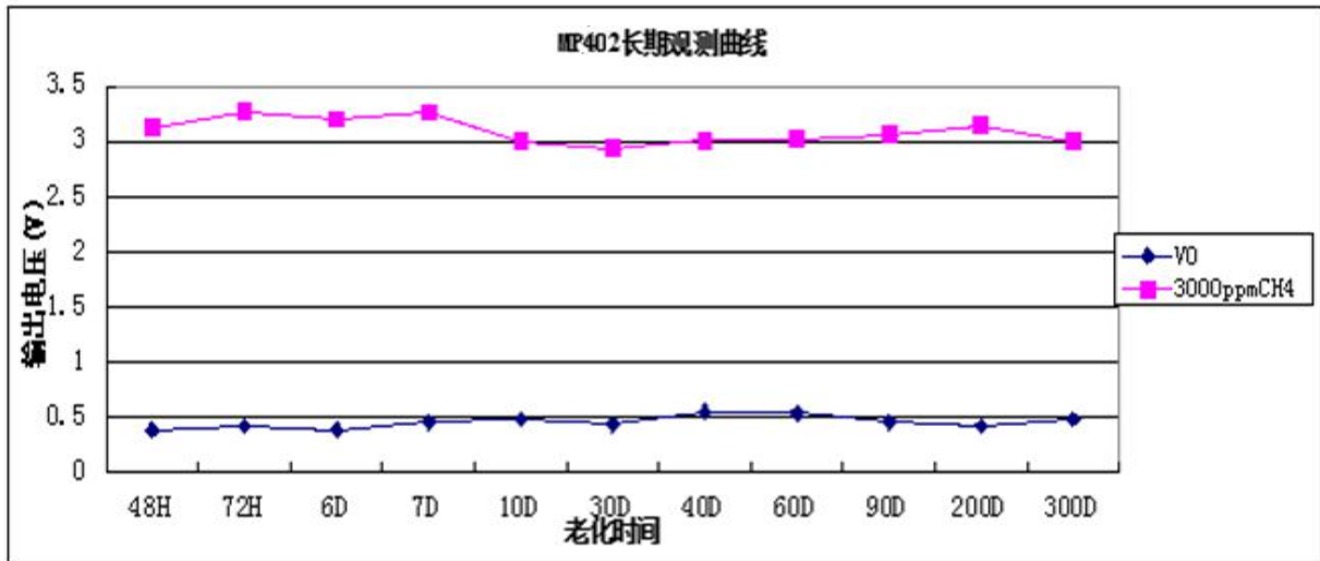
图 7: 长期稳定性曲线
